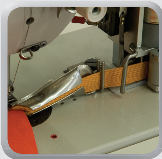
Motorisch angetriebene, spannungsgesteuerte Bandzuführung.
