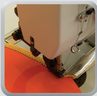
Die Umlage des Bandes erfolgt unmittelbar vor der Nadel. Dadurch sind selbst kleinste Radien problemlos einzufassen.
